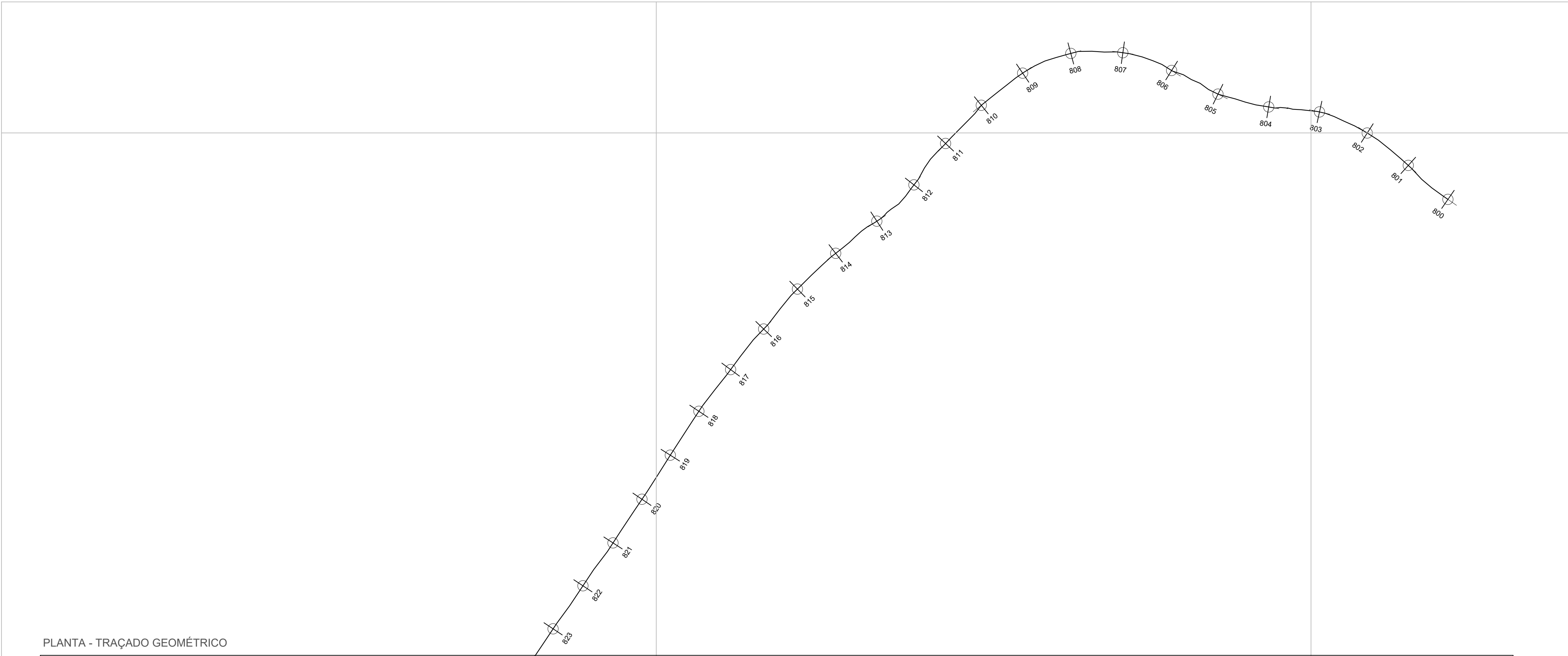
PLANTA - TRAÇADO GEOMÉTRICO
