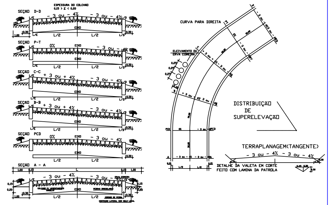
SEÇÃO TRANSVERSAL
